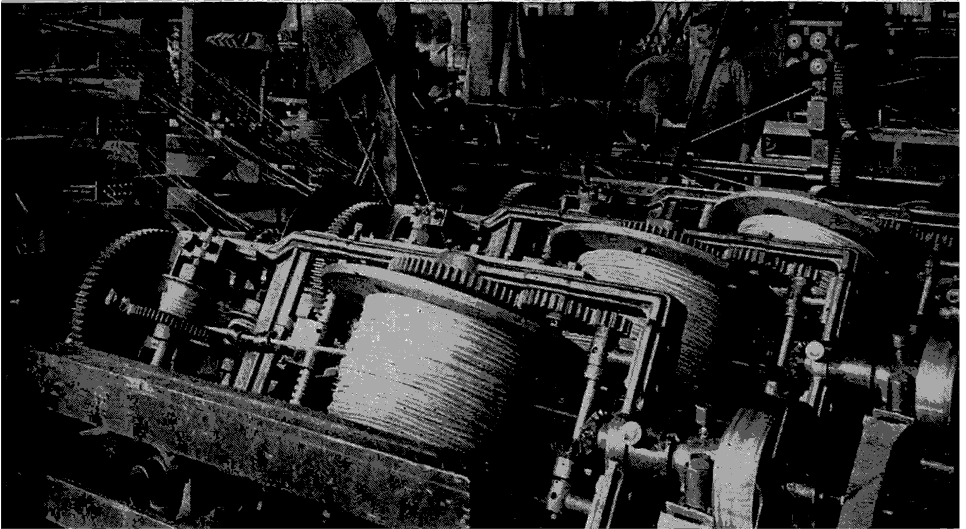
ခေတ်မှီကြိုးစက်ရုံ၏ အတွင်းပိုင်းရှုခင်းတစ်ခုကိုမြင်ရပုံ
