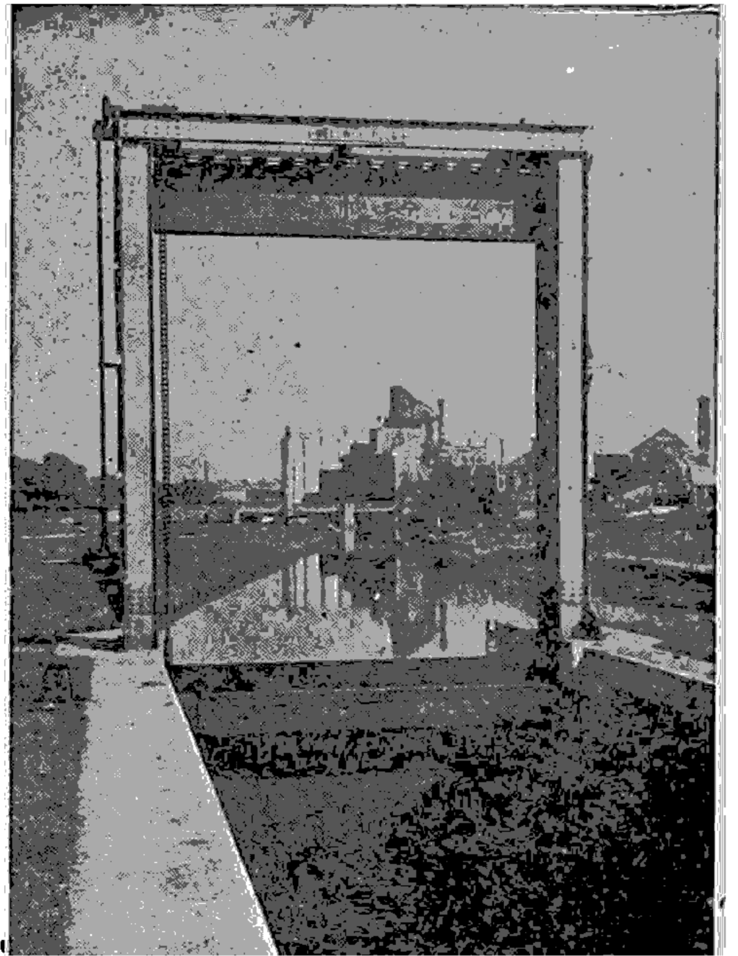
အချို့ ရေပြင်ညှိ ဆည်တို့တွင် ရေသွင်း ရေထုတ်ရန် တံခါးကို အေးတိုက် အဖွင့်မဟုတ်ဘဲ စက်သီးကြိုးဖြင့် ဆွဲကာ အတင်အချ ပြုလုပ်ရန် စီစဉ်ထားသည်။
