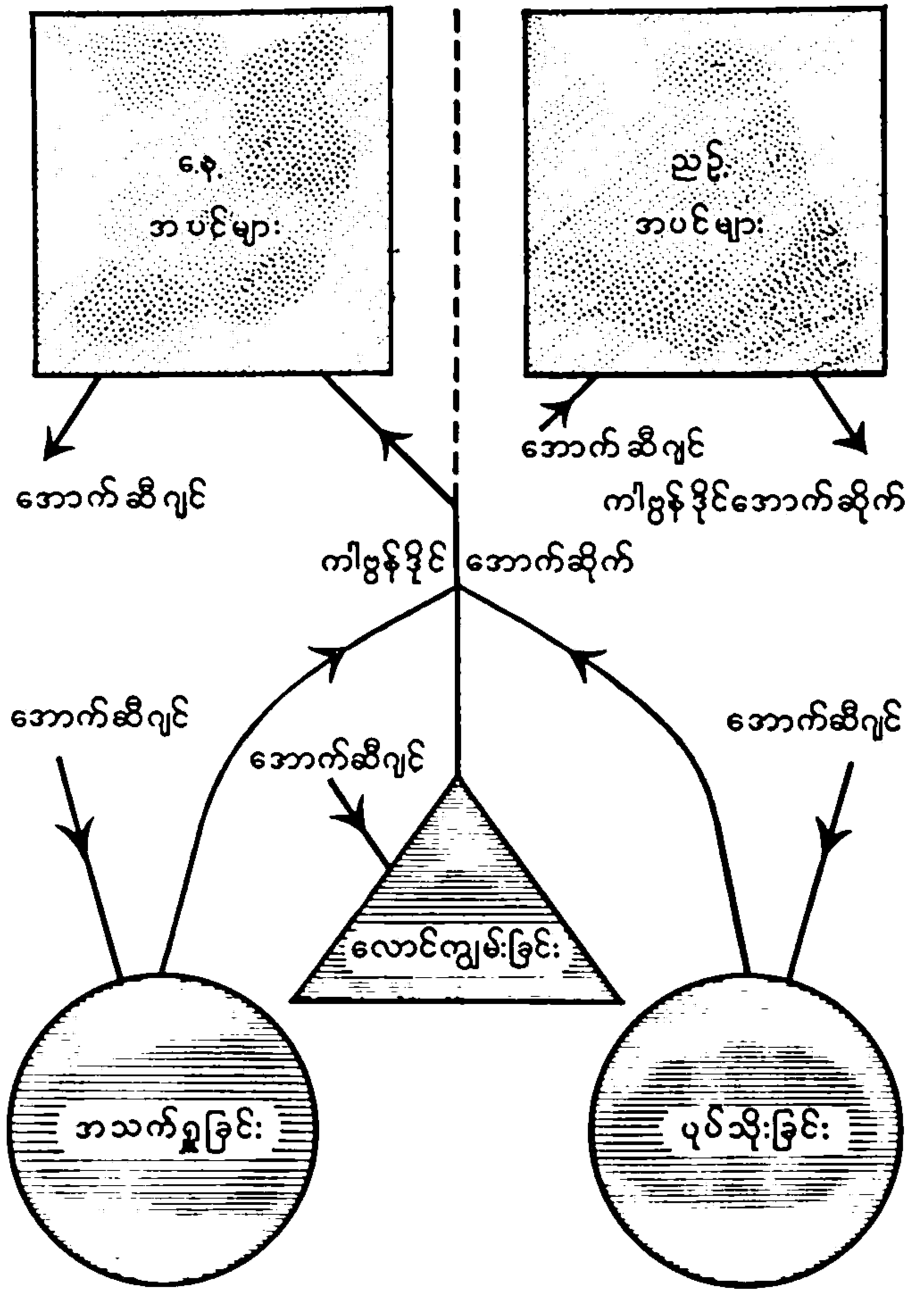
ပတ်ဝန်းကျင်လေထဲ၌ ကာဗွန်ဒိုင်အောက်ဆိုက် တည်ရှိပုံ အသက်ရှူခြင်း၊ လောင်ကျွမ်းခြင်း၊ ပုပ်သိုးခြင်းနှင့် ညှို့ဖက်အပင်တို့သည် ကာဗွန်ဒိုင်အောက်ဆိုက် အဆိပ်ဓါတ်ငွေ့ကို ထုတ်ပေးကြ၏။ သို့သော် ထိုဓါတ်ငွေ့ကို နေရောင်ရသော နေဖက်တွင် အပင်များက အသုံးပြုခြင်းဖြင့် လေကို သန့်ရှင်းစေပြန်သည်။
