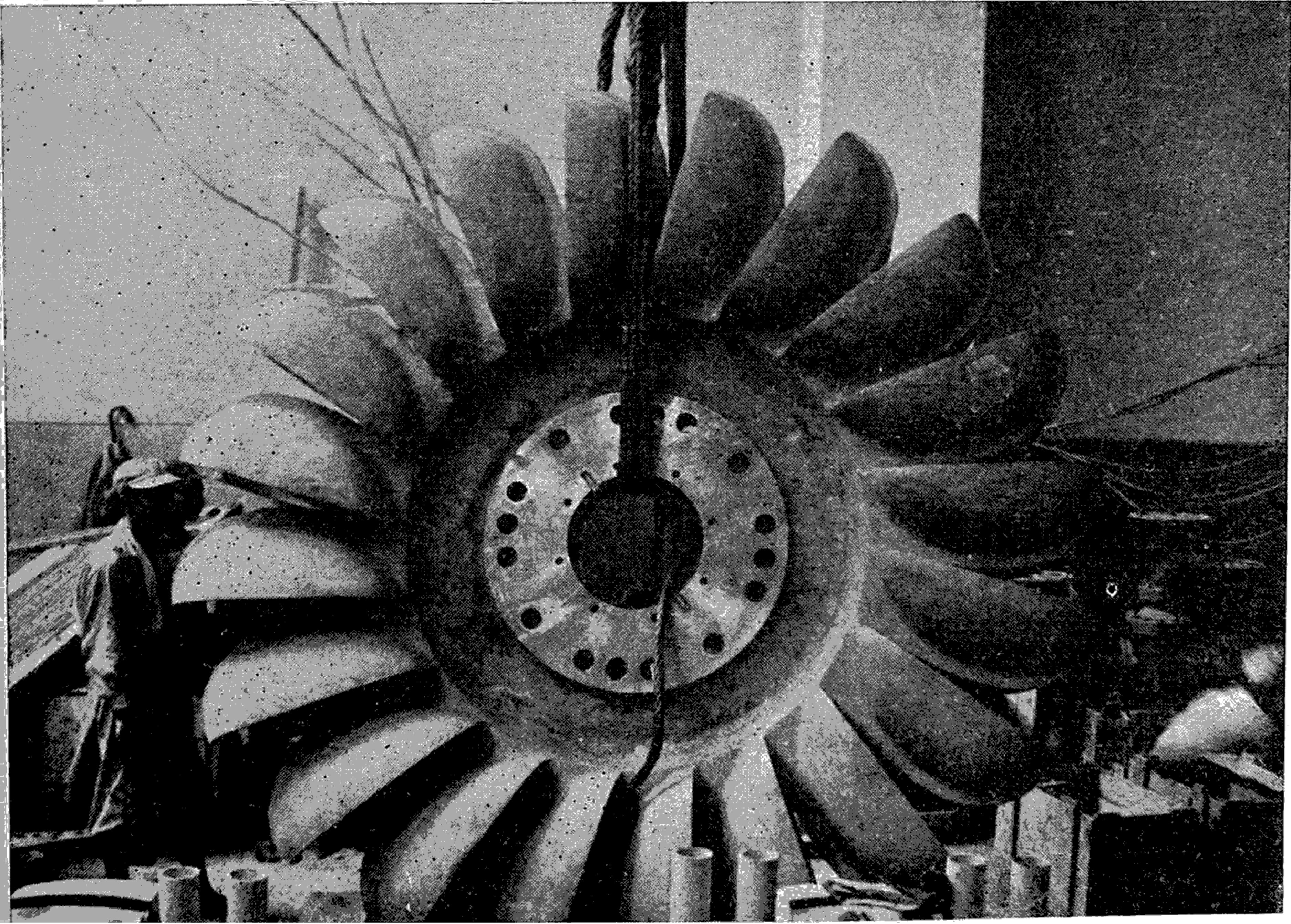
ရေအားမှ လျှပ်စစ်ဓာတ်အားအဖြစ်သို့ ပြောင်းလဲပေးမည့် ရေရဟတ်ကြီးတင် ခွက်ကြီးများ ပါရှိသည်။ ပန်းထွက်လာသော ရေအဟုန်သည် ထိုခွက်ကြီးများကိုအရှိန်ပြင်းစွာ တွန်းသဖြင့် ရဟတ်ကြီး လည်ရခြင်းဖြစ်သည်။
