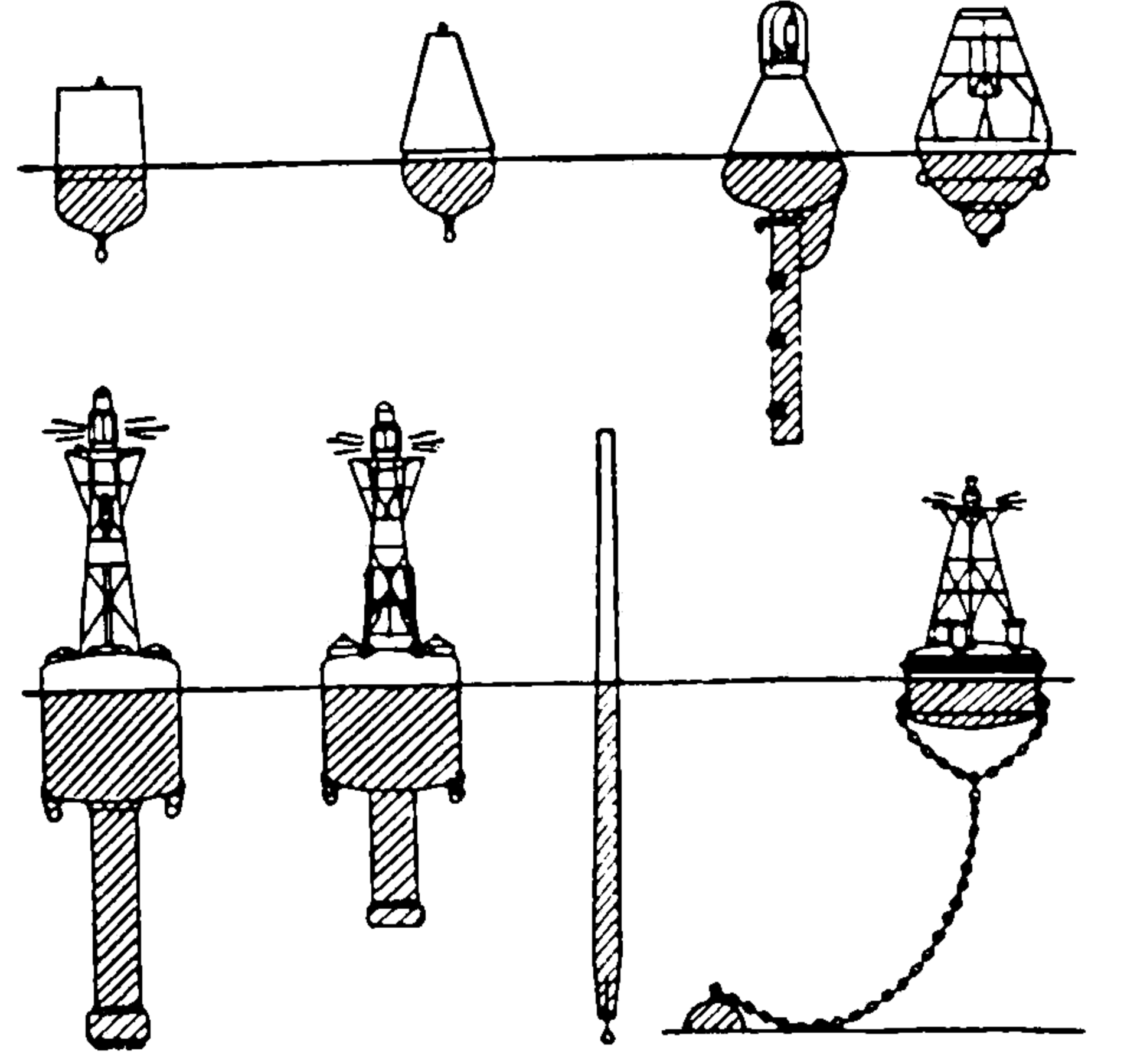
အပေါ် (ဝဲ) ရိုးရိုးဗော်ယာ ၂ မျိုးနှင့် (ယာ) ခေါင်းလောင်းတပ် အချက်ပေး ဗော်ယာ ၂ မျိုးတို့ဖြစ်ကြသည်။ အောက်ပုံများမှာမူ မီးပြဗော်ယာများ ဖြစ်ကြသည်။
