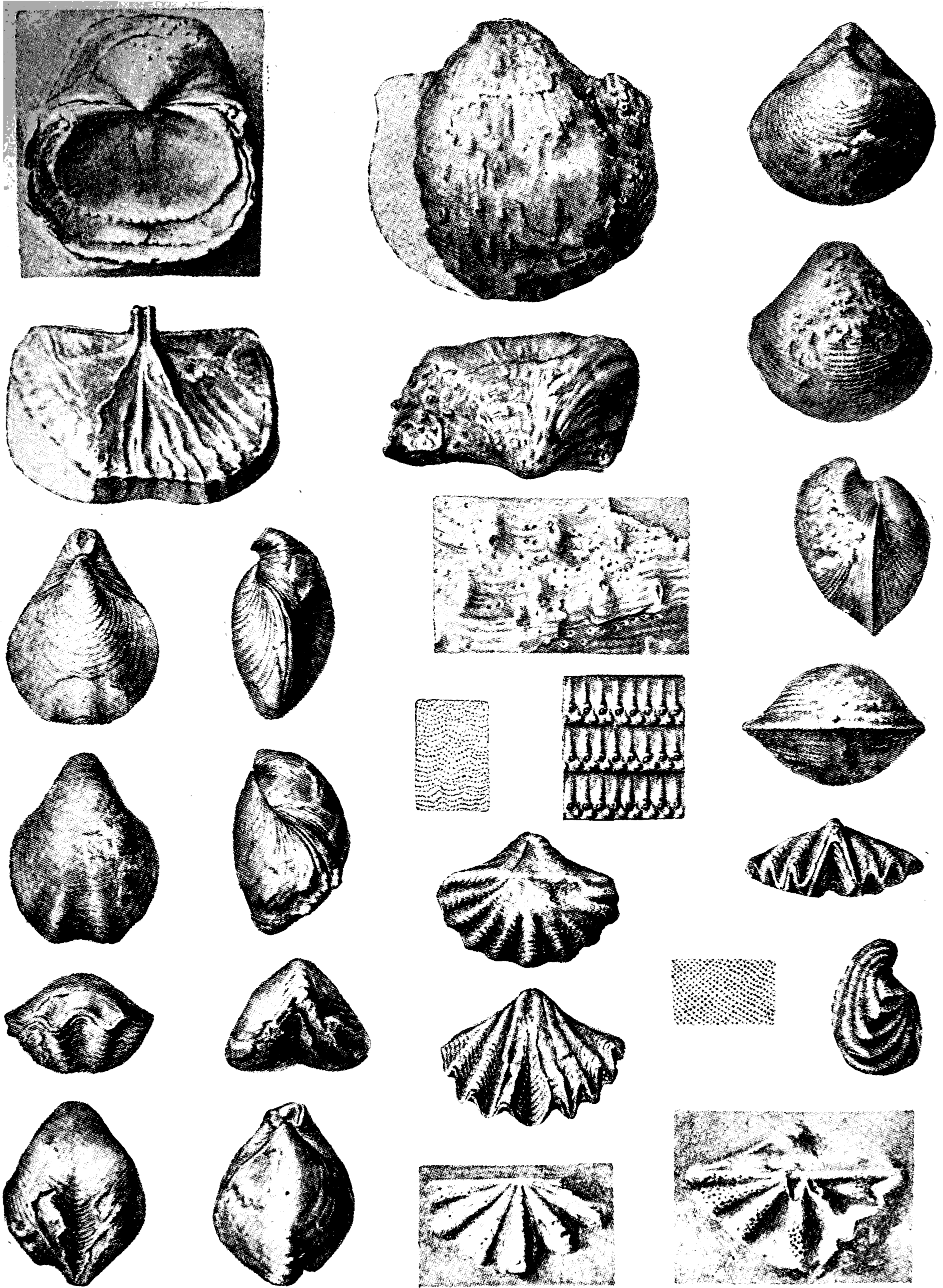
လွန်ခဲ့သော နှစ်ပေါင်း သန်း ၃၀၀ ခန့်က ဖြစ်ပေါ်ခဲ့သော ရှမ်းပြည်တောင်ပိုင်းရှိ ကုန်းပြင်မြင့် ထုံးကျောက်လွှာများမှ ရရှိသော ရုပ်ကြွင်း ကျောက်များပုံဖြစ်သည်။ ယင်းကို လေ့လာသောပညာကို နိဒါတက ဗေဒ ဟု ခေါ်သည်။
