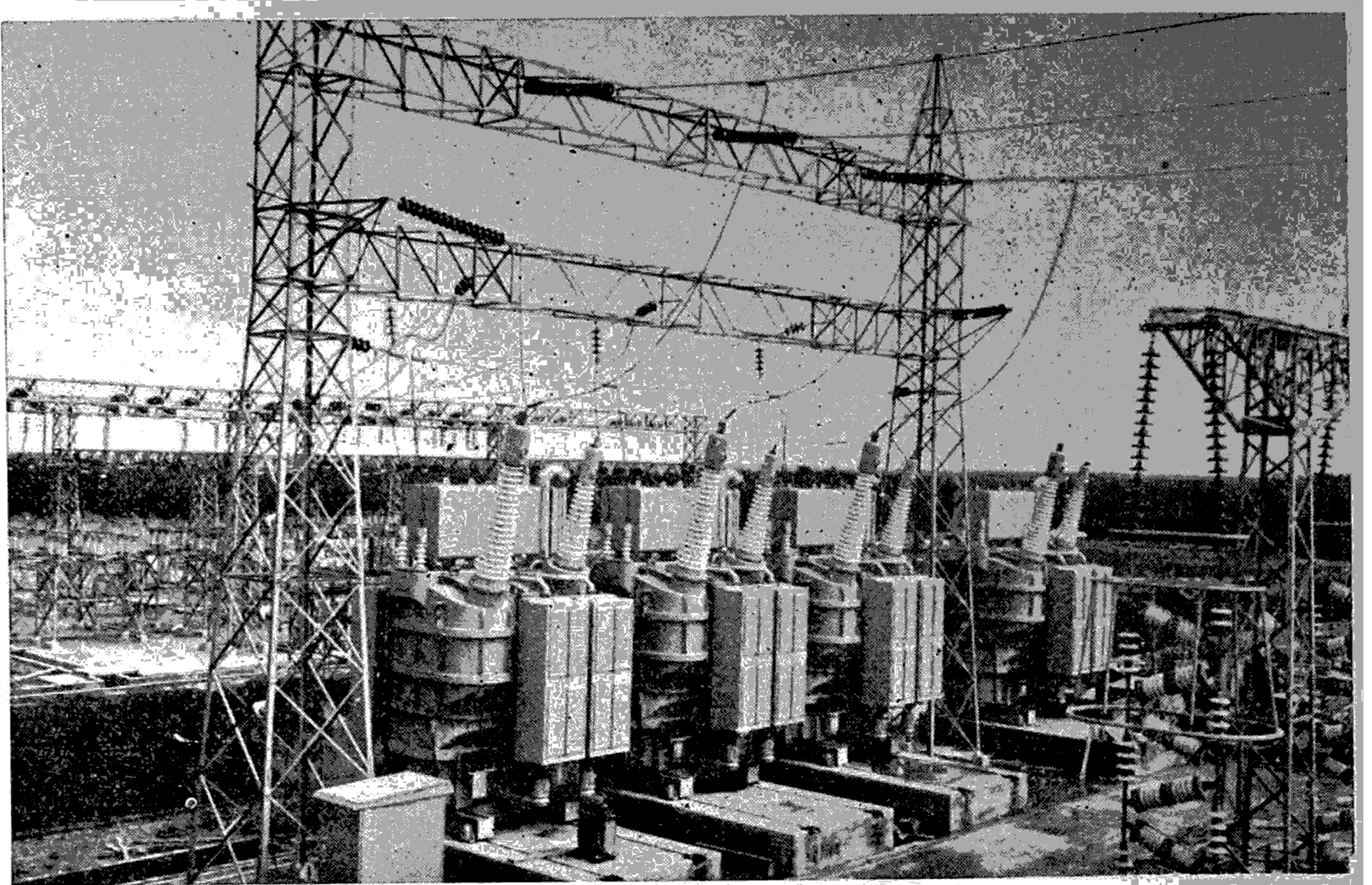
လောပီတမုရရှိသော လျှပ်စစ်ဓာတ်များကို တဆင့်ပို့ပေးရသော ကေဗီ၊ အေ ၆၀,၀၀၀ အားရှိသည့် ဓာတ်အားဖြန့်စက်ကြီး
