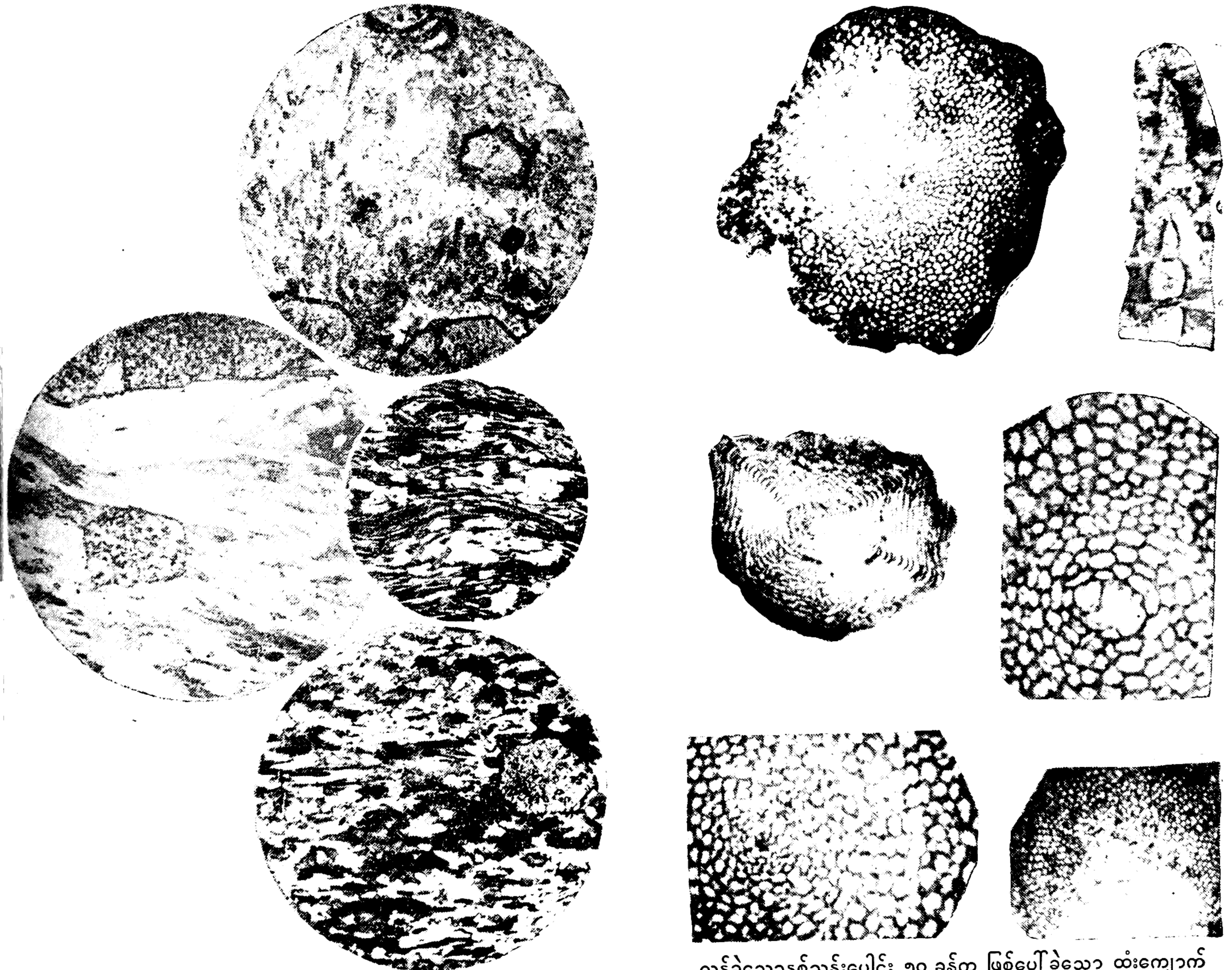
ကျောက်ဆည်တောင်ပေါ်ရှိ ဝေဘူကျောက်ကို ပါးပါးလွှာလွှာ ဖြတ်ထားပြီး၊ မိုက္ကရိုစကုပ်အောက်တွင် ကြည့်သောအခါ တွေ့မြင်ရသည့် ဝေဘူကျောက် ဖြတ်ပိုင်းပုံ။ ဤပညာကို သေလဗေဒ ဟုခေါ်သည်။
