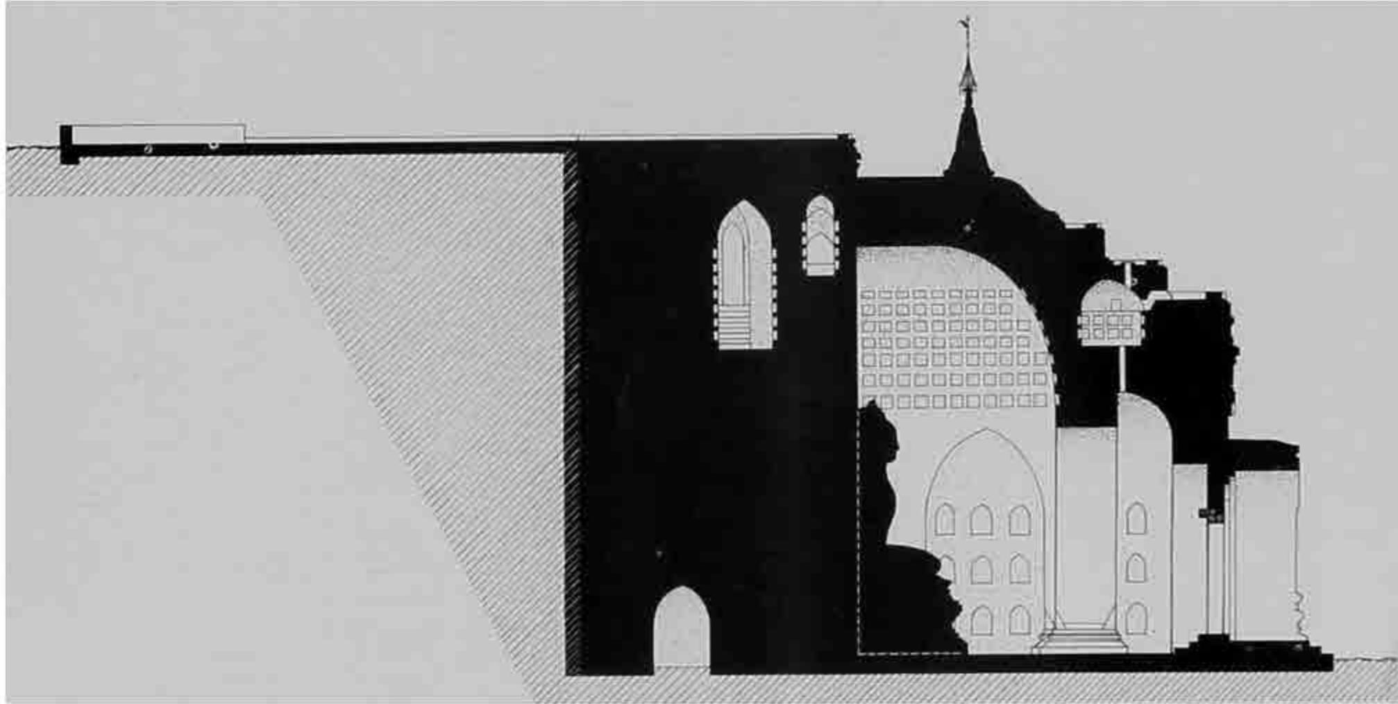
ကျောက်ဂူဥပင်ဖြတ်ပိုင်းပုံ
